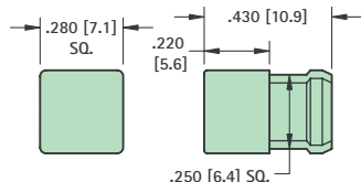
FIG. 5 T-1 3/4
