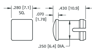
FIG. 7 T-1 3/4
