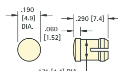
FIG. 3 T-1
