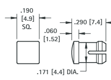
FIG. 6 T-1
