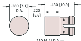
FIG. 2 T-1 3/4
