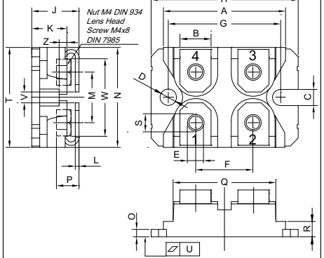
X027a SOT-227 B miniBLOC Weight = 29 g X027b SOT-227 UI miniBLOC
