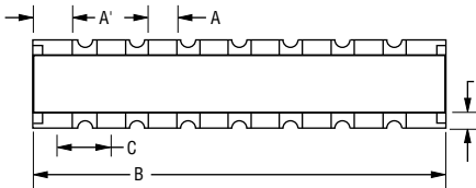
CAY16-J8
