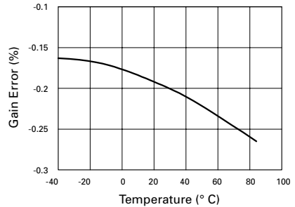
NEG Gain Error V Temp.
