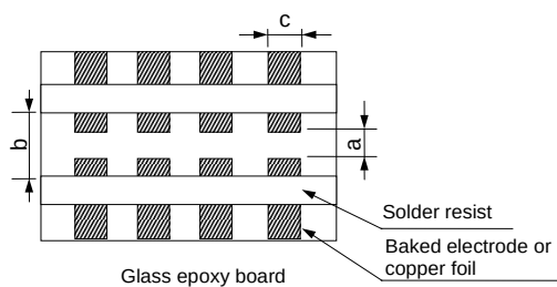
Fig.3 (in:mm)
