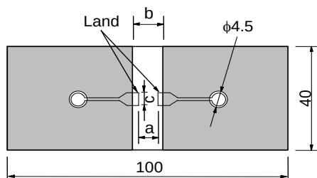
Fig.1 (in:mm)
