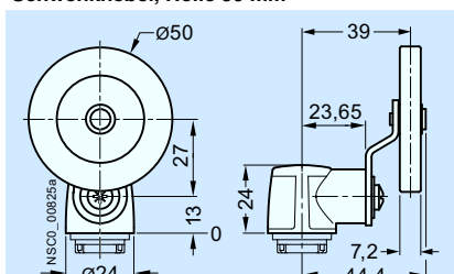
Schwenkhebel, Rolle 50 mm
