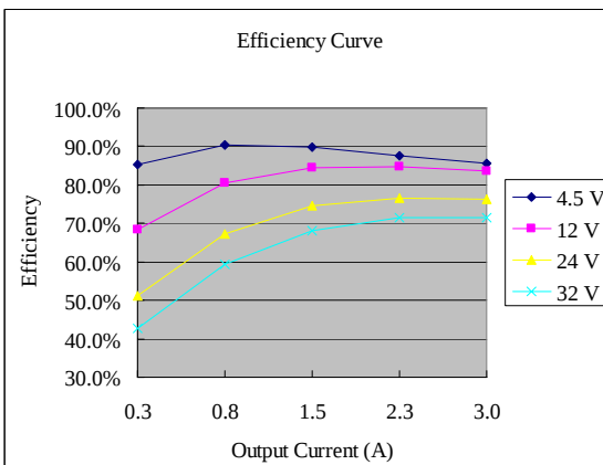
Vo=1.5 V
