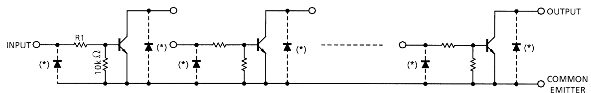
TD62504P / F
