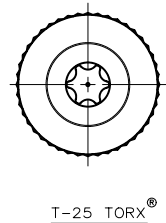
T-25 TORX®
