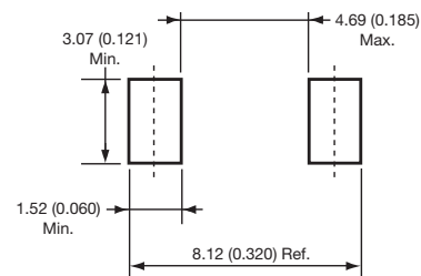
DO-214AB (SMC)
