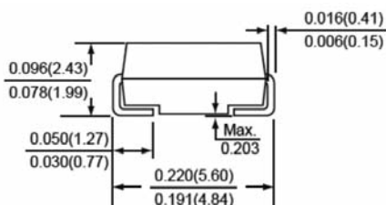
SMA/DO-214AC
