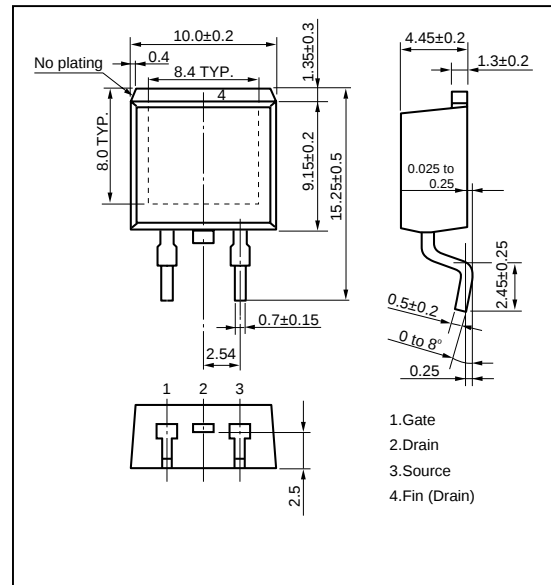
2)TO-263 (MP-25ZK)
