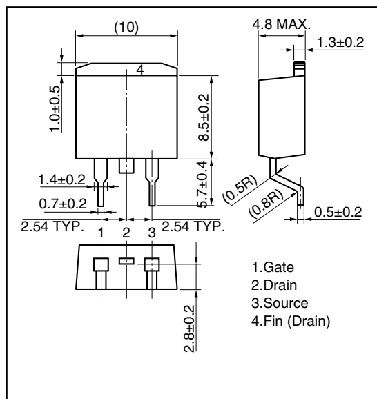
3)TO-263 (MP-25ZJ)
