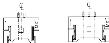
ロック形状図 LOCK CONFIGURATION
