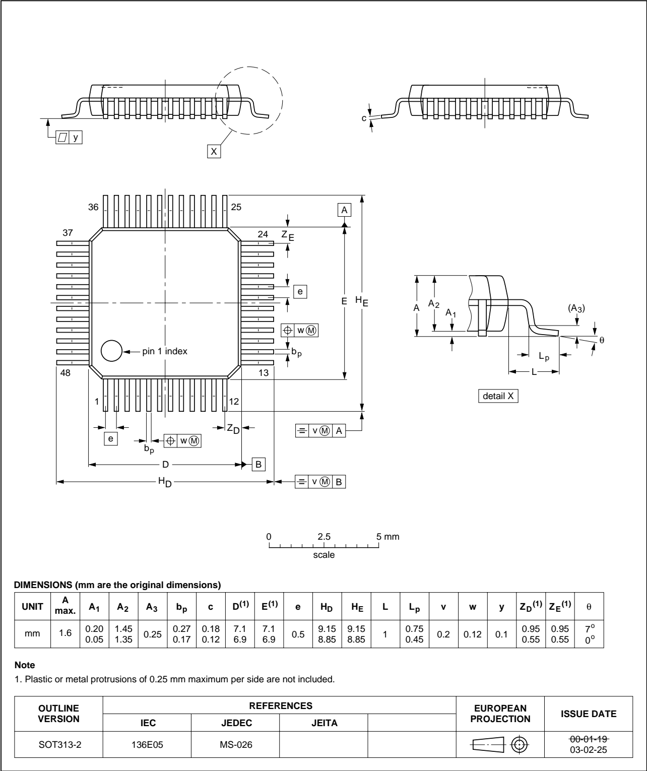
Fig 7. SOT313-2
