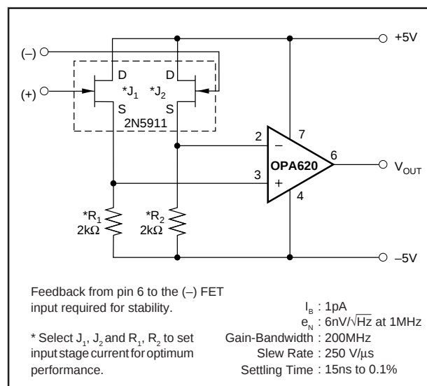
FIGURE 13. Low Noise, Wideband FET Input Op Amp.
