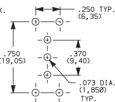
E101MD1_BE SPDT
