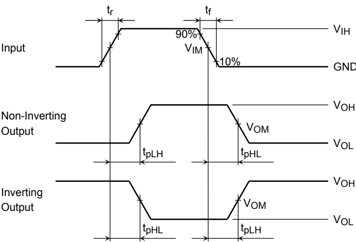
図 2 t_{pLH} , t_{pHL}
