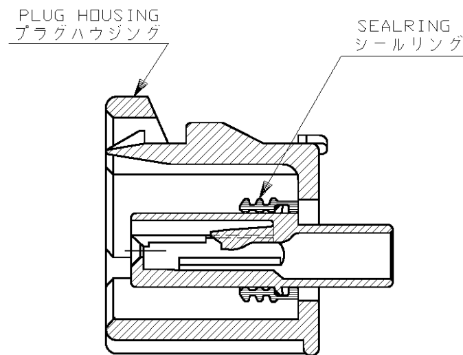
SECT 断面 A-A
