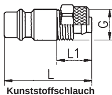
Kunststoffschlauch
