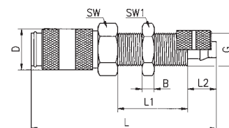
Schottverschraubung für Kunststoffschlauch
