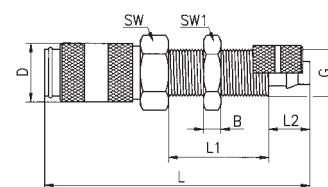
Schottverschraubung für Kunststoffschlauch
