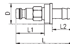
Schlauchanschluß
