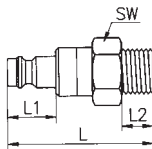
Außengewinde
