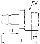
Innengewinde
