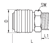
Außengewinde
