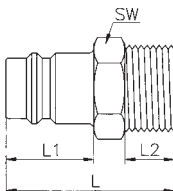
Außengewinde
