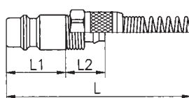
Knickschutzfeder
