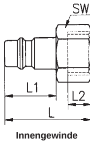
Innengewinde
