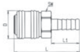
Schlauchanschluß
