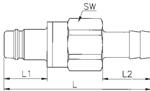
Schlauchanschluß
