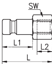
Innengewinde
