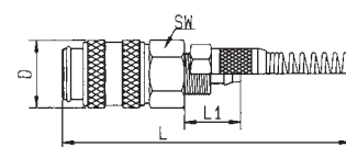
Knickschutzfeder
