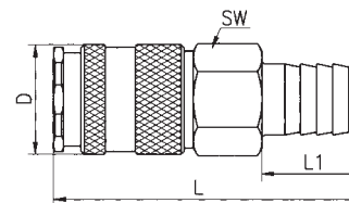
Schlauchanschluß
