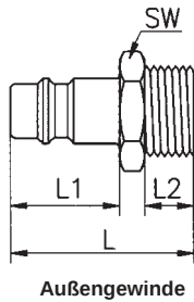
Außengewinde
