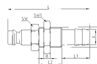
Schott-Stecktülle für Schlauchanschluss
