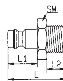
Außengewinde
