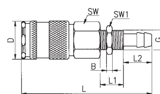
Schottverschraubung für Kunststoffschlauch
