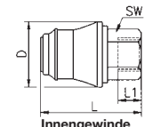
Innengewinde
