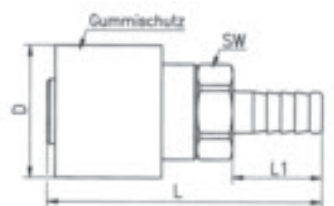
Schlauchanschluß
