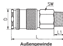
Außengewinde
