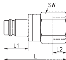
Innengewinde
