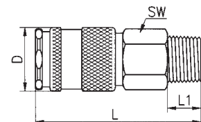
Außengewinde
