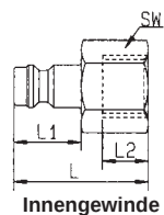
Innengewinde
