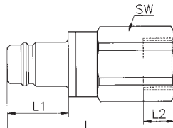
Innengewinde
