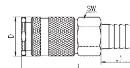
Schlauchanschluß
