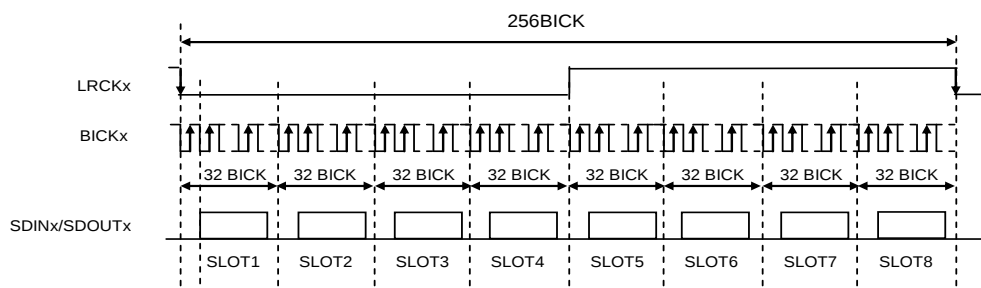
Figure 34. TDM Mode I 2 S Compatible (BICK=256fs)
