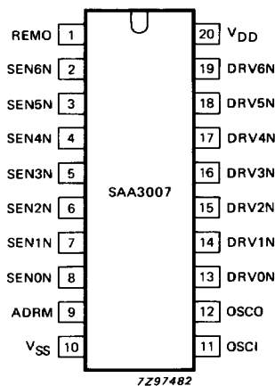
Fig. 2 Pinning diagram.
