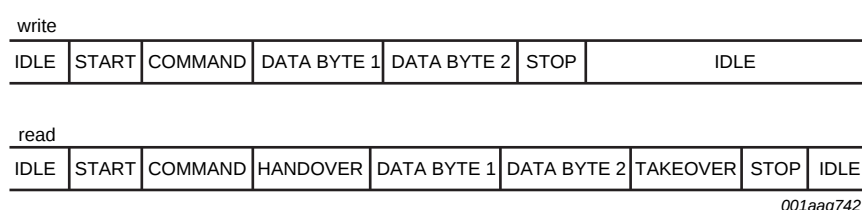
Fig 12. OWI data format
