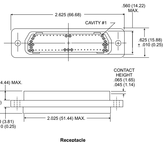
Receptacle
