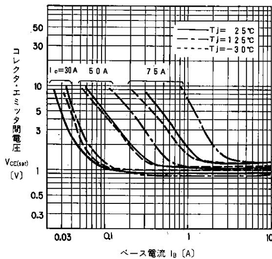
出力特性
