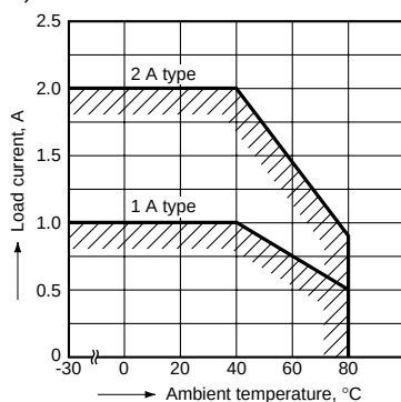
1-2. Load current vs. ambient temperature (ODC)
