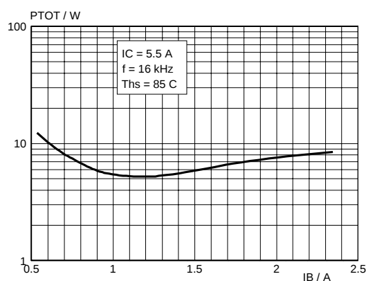
Fig.9. Limit P_{TOT} ; T_{HS} = 85^\circ\text{C} P_{TOT} = f(I_{B(end)}) ; I_C = 5.5\text{ A} ; f = 16\text{ kHz}
