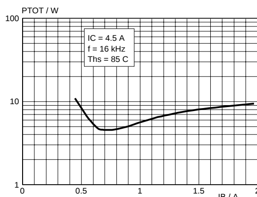
Fig.8. Limit P_{TOT} ; T_{HS} = 85^\circ\text{C} P_{TOT} = f(I_{B(end)}) ; I_C = 4.5\text{ A} ; f = 16\text{ kHz}
