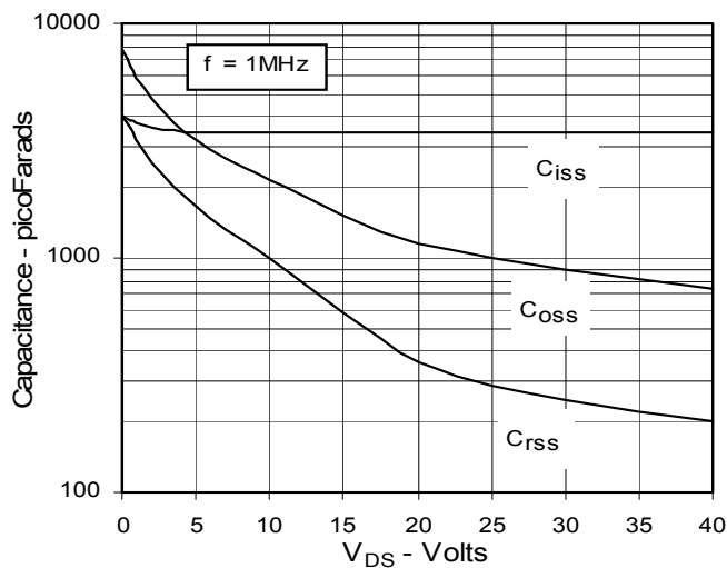
Fig. 11. Capacitance
