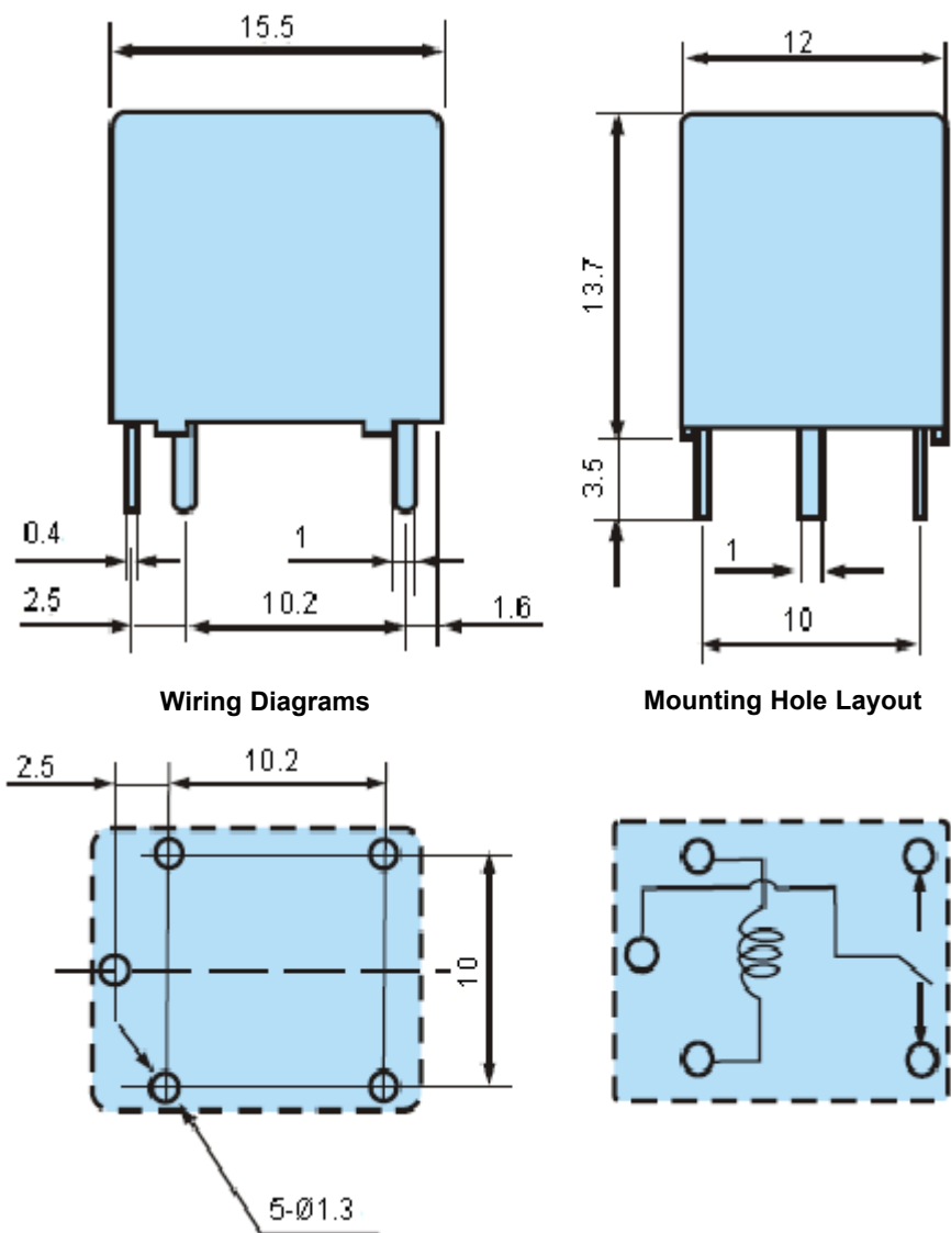
Dimensions : Millimetres
