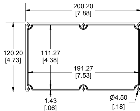
Lid
