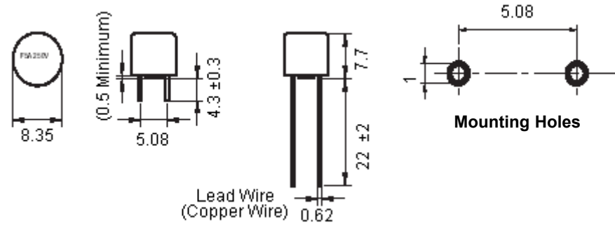
Dimensions : Millimetres
