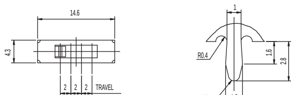
K DETAIL 2:1
