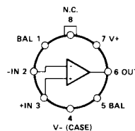
TO-99 (J-Suffix)
