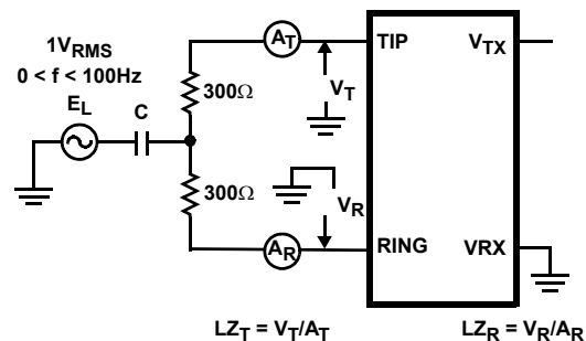
FIGURE 2. LONGITUDINAL IMPEDANCE
