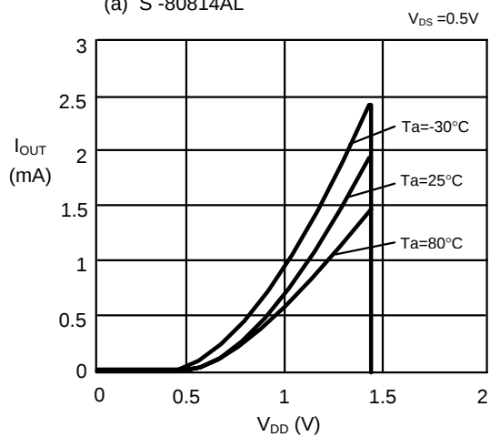
(a) S-80814AL
