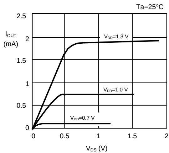
(a) S-80814AL
