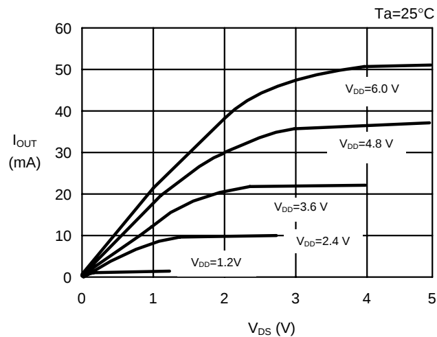
(b) S-80860AL
