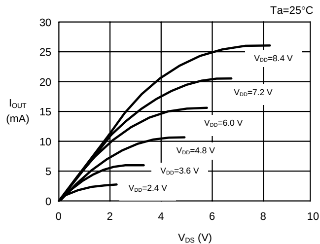
(b) S-80815AL
