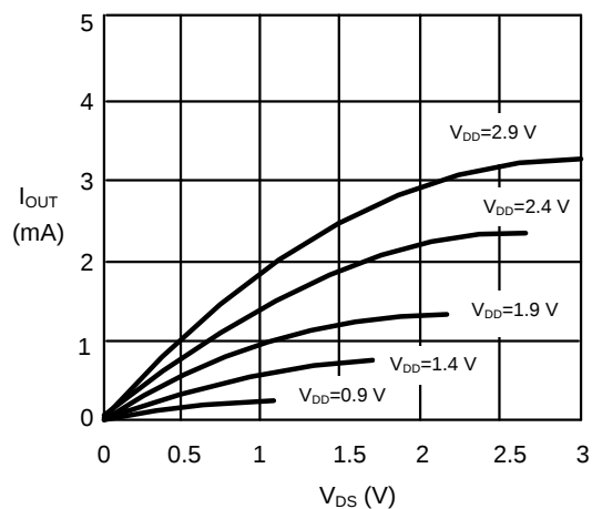
(a) S-80808AL
