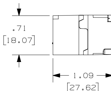
COUPLER MODULE
