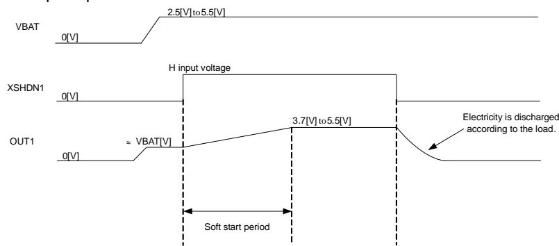
(d) PWM/PFM
