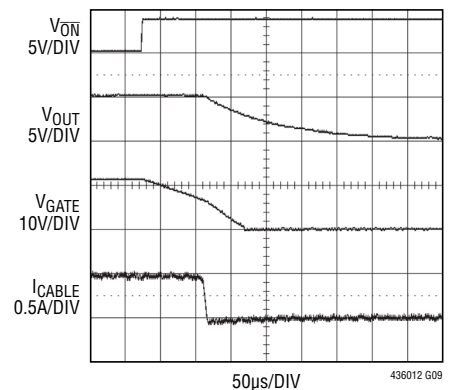
Entering Sleep Mode (LTC4360-1)
