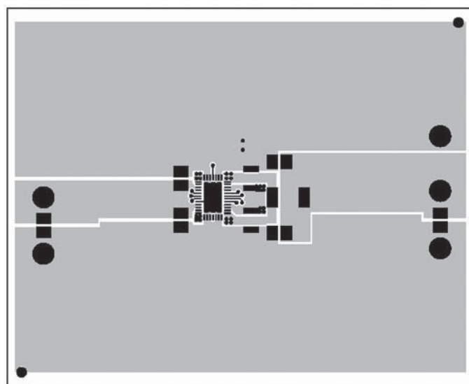
Top Layer
