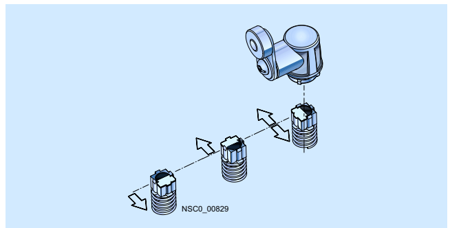
Schwenkantrieb für Schwenk- und Stangenhebel mit Einstellung der Schaltrichtung rechts, links oder rechts/links (Standard für alle Schwenkantriebe außer Gabelhebel)
