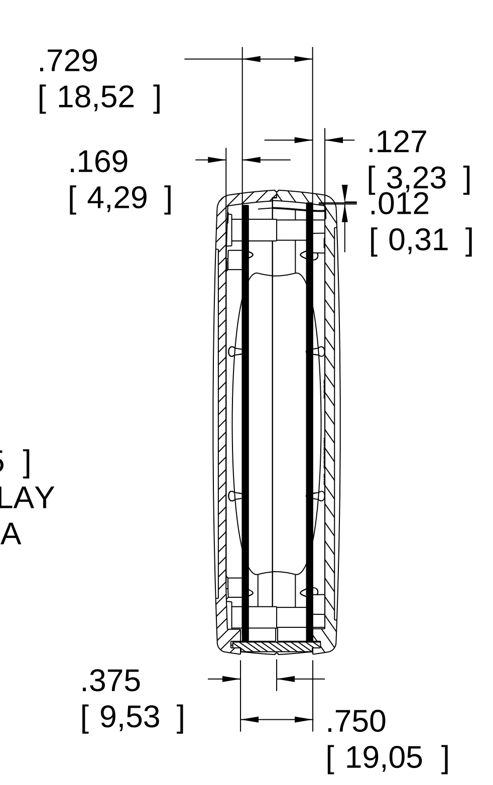
SECTION A-A
