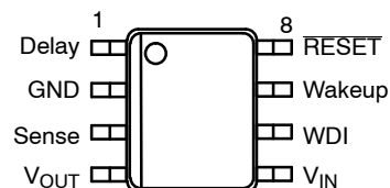
SO-8 EP
