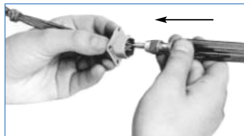
Démontage contacts/ Contact extraction/Abziehen der Kontakte
