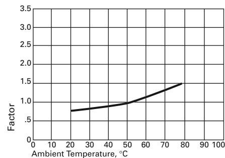
AQB-LF100 BREAKERS
