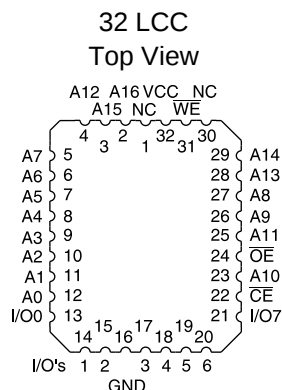
NC 1 32 VCC A16 2 31 WE A15 3 30 NC A12 4 29 A14 A7 5 28 A13 A6 6 27 A8 A5 7 26 A9 A4 8 25 A11 A3 9 24 OE A2 10 23 A10 A1 11 22 CE A0 12 21 I/O7 I/O0 13 20 I/O6 I/O1 14 19 I/O5 I/O2 15 18 I/O4 GND 16 17 I/O3
