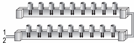
1. alimentación 12VDC 2. masa 0V
