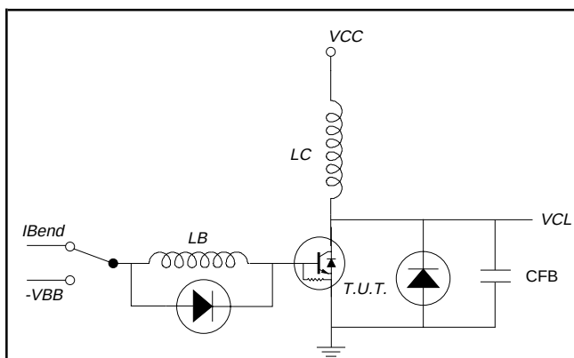
Fig.13. Test Circuit RBSOA. V_{CC} = 150\text{ V} ; -V_{BB} = 1 - 4\text{ V} ; L_C = 1\text{ mH} ; V_{CL} = 1500\text{ V} ; L_B = 1 - 3\text{ }\mu\text{H} ; C_{FB} = 1 - 4\text{ nF} ; I_{B(end)} = 0.8 - 4\text{ A}
