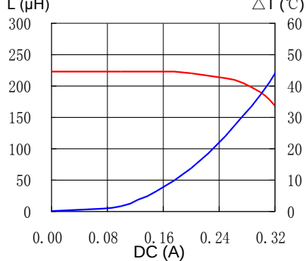
25. CDC5D23BNP-221KC
