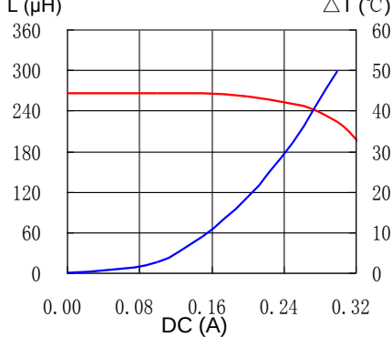
26. CDC5D23BNP-271KC
