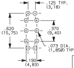
7201J1__BE2 DPDT
