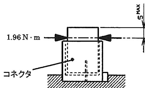
Fig.8 こじり耐久性
