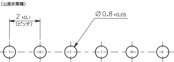
基板穴推奨寸法
