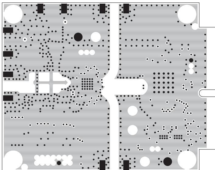
Inner Layer 2
